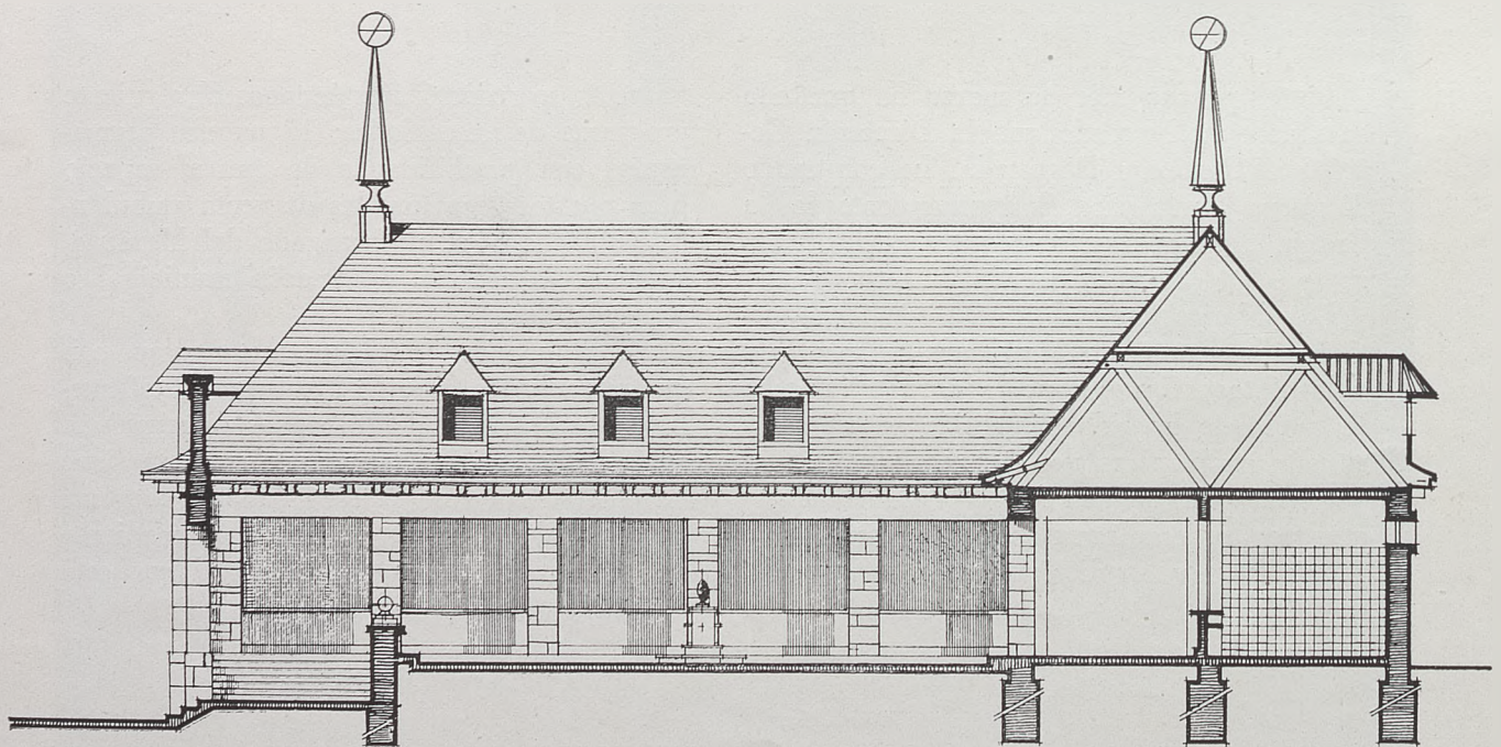
Sección A-B.
