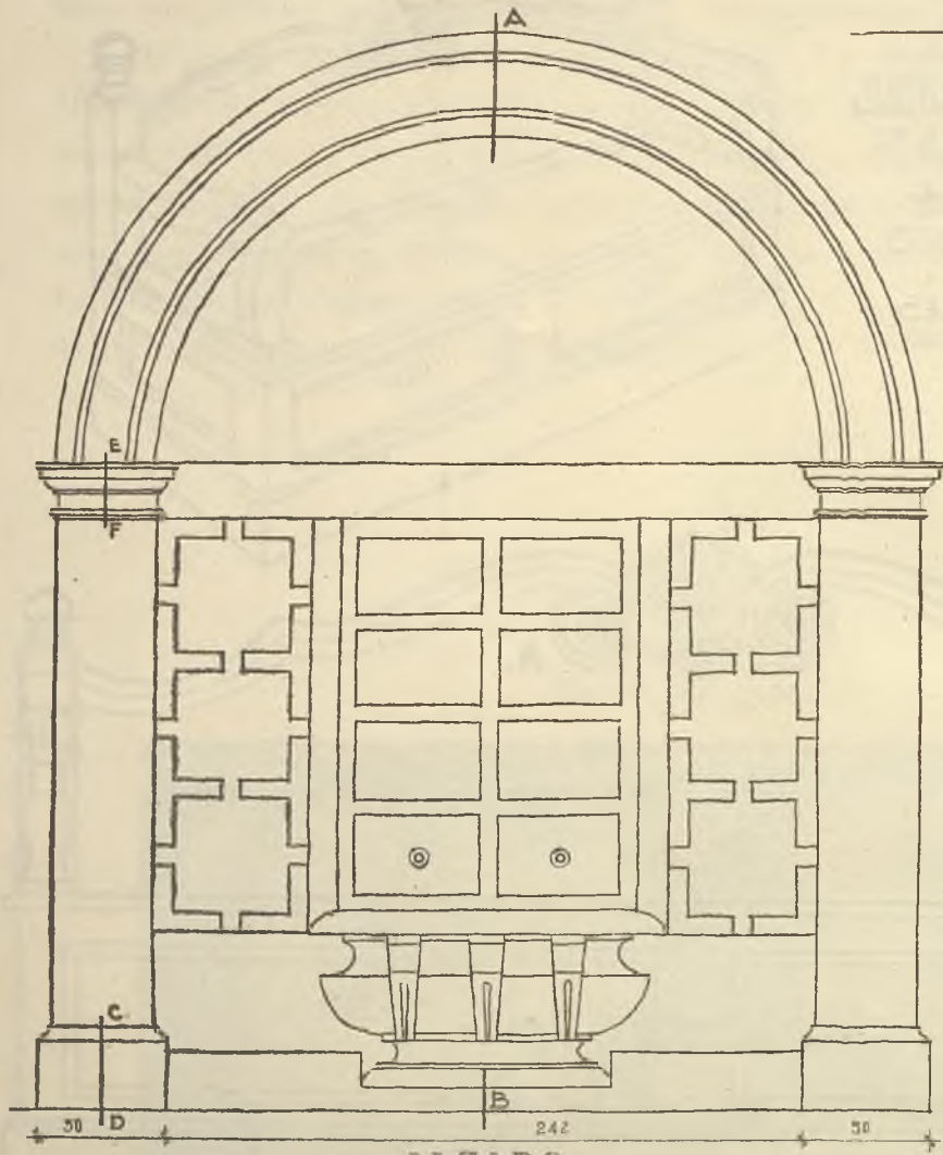
ALZADO
