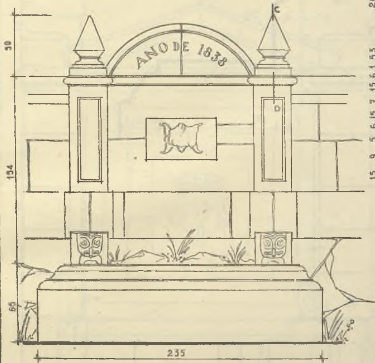
ALZADO
