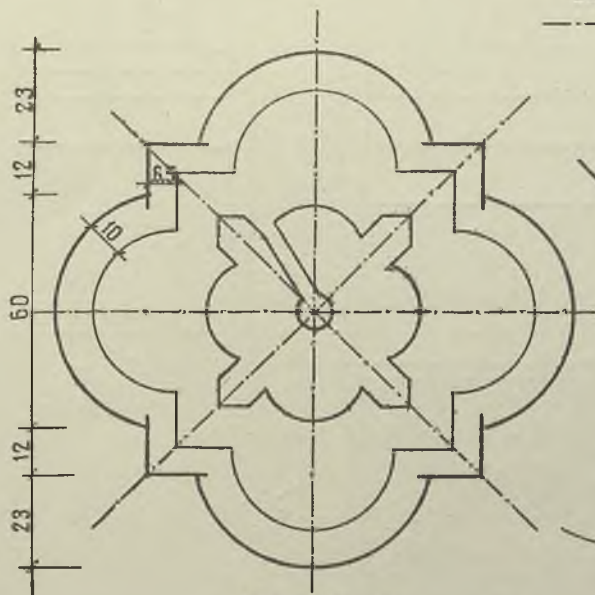
PLANTA - H
