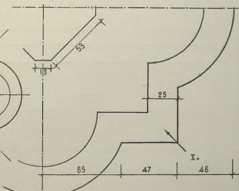
PLANTA
