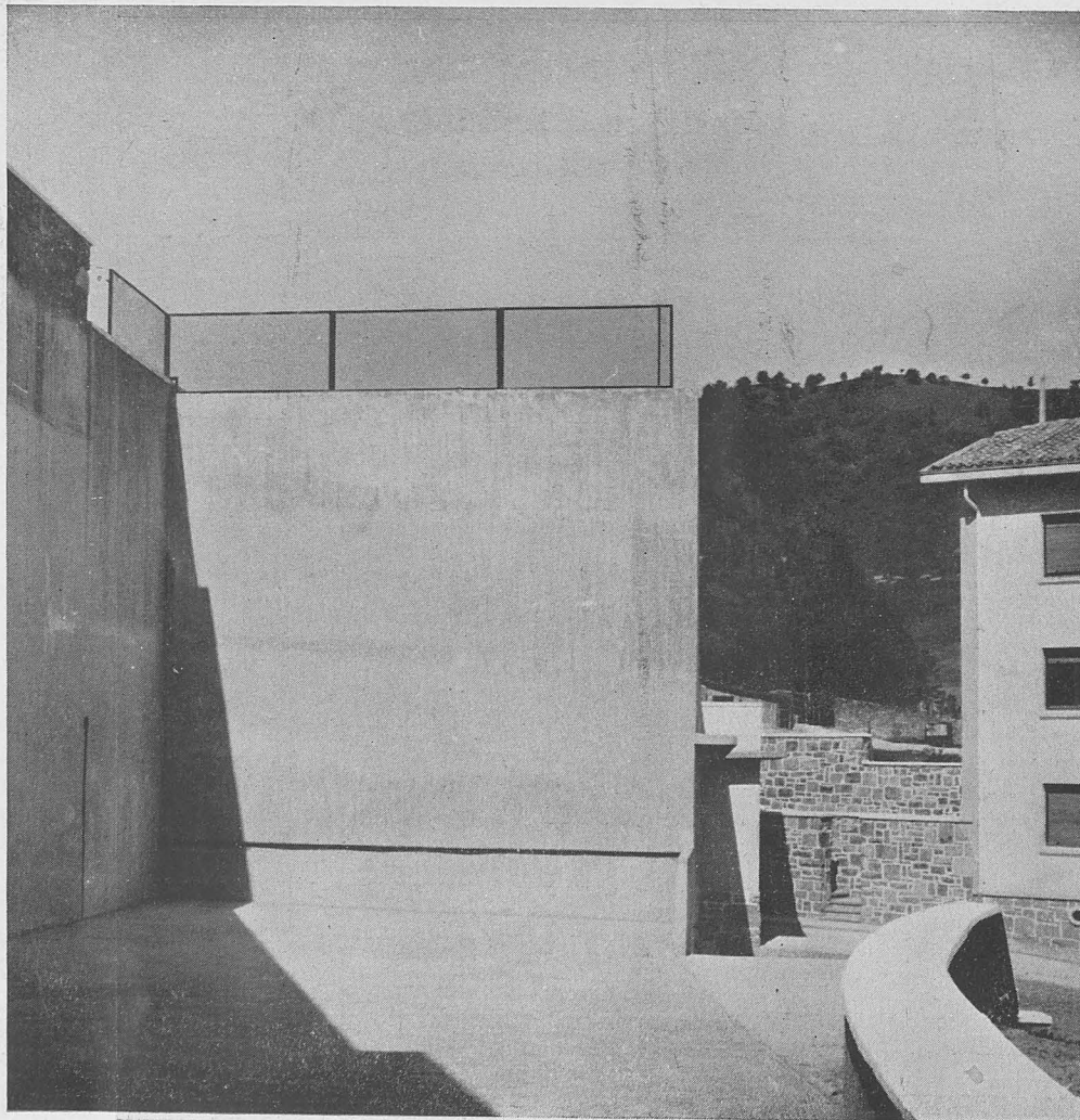
Frontón. Detalles.
