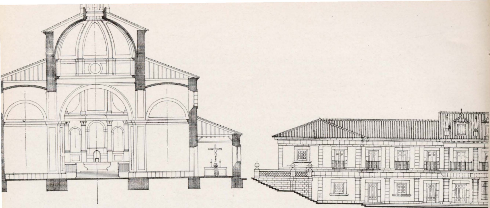
Alzado de conjunto de la plaza Mayor
