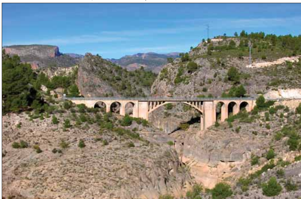
Puente del embalse de la Fuensanta, en el término municipal de Yeste, Albacete.
