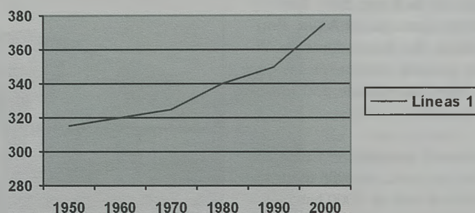
Concentraciones atmosféricas de dióxido de carbono, 1958-98.
