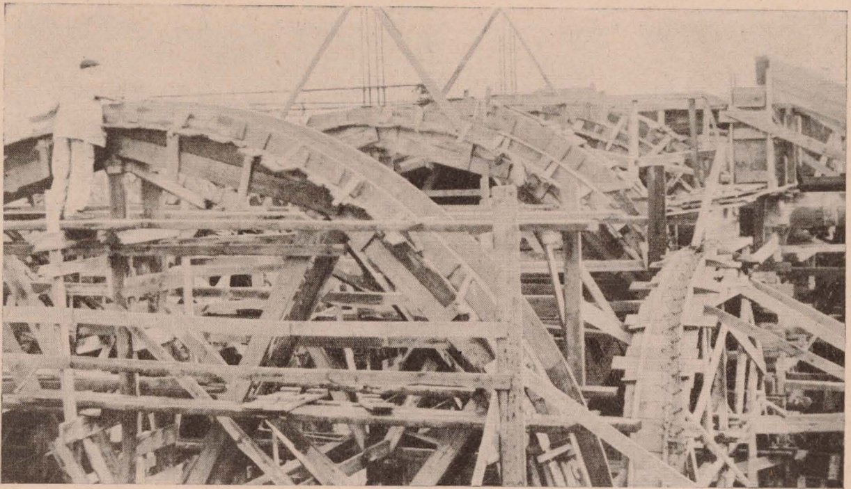
Gatica : Obras de reconstrucción de la Iglesia parroquial. Abajo. Durango : La Iglesia, antes y después de su reconstrucción. Fotos comparativas.
