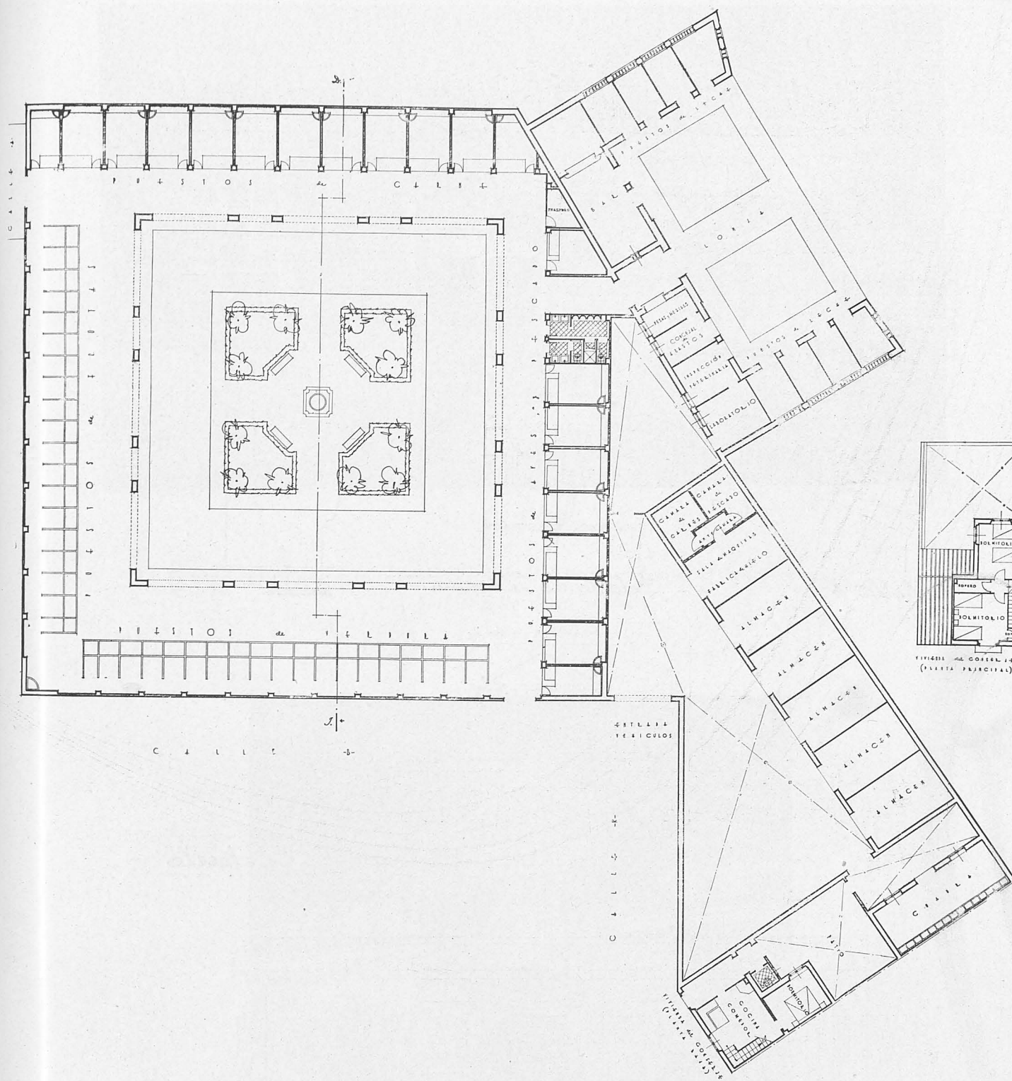
MARMOLEJO.—Jaén. Mercado de Abastos. Planta general.
