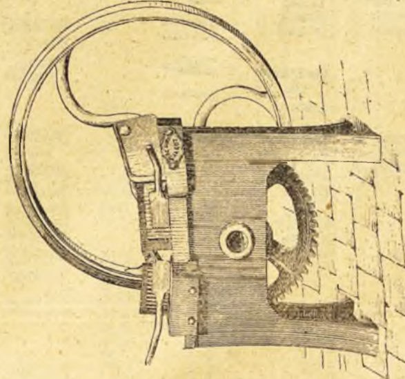
Máquina de recalcar
