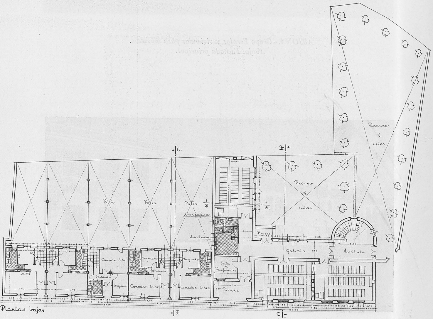
ARJONA.-Grupo Escolar y viviendas para maestros, Plantas.
