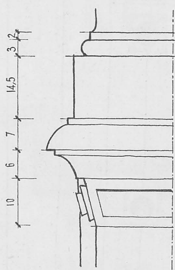
PERFIL A-B.
