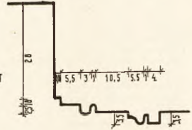
SECCION M-N
