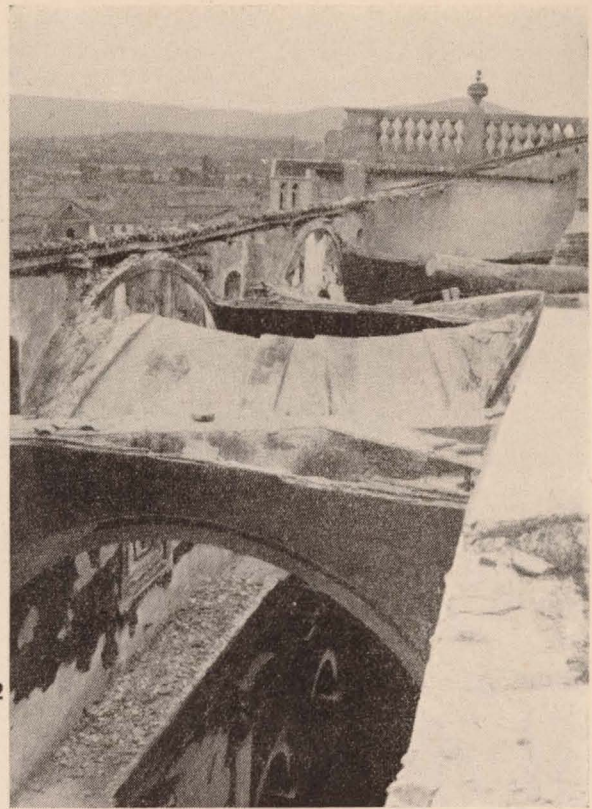
1, 2 y 3. Estado en que quedó la Catedral de Vich, antes de empezar los trabajos de reconstrucción.— 4. Plataforma-andamiaje, construida al nivel de la cornisa del templo, y andamiaje para el refuerzo de los arcos, sostén de las bóvedas.
