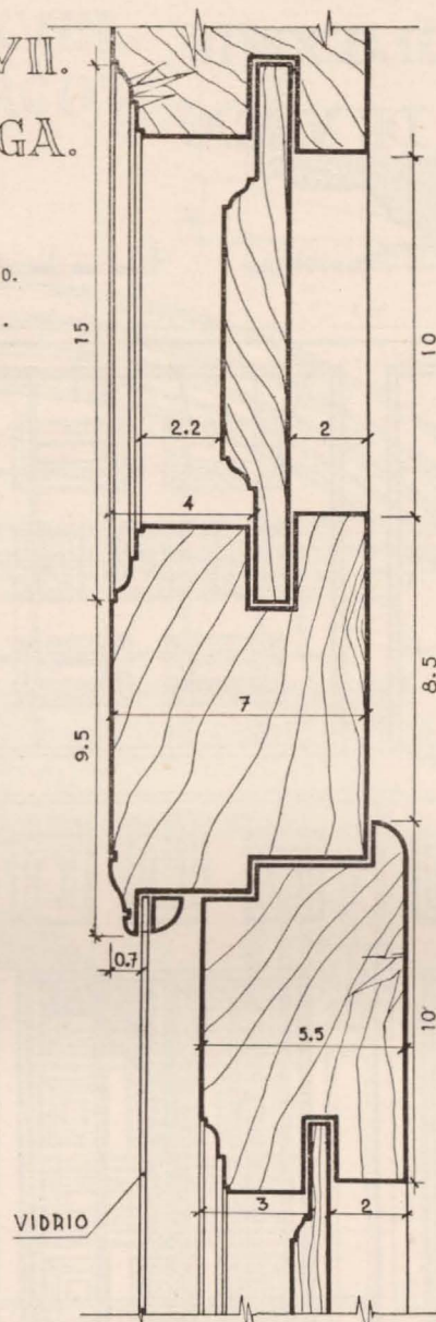
SECCION A-B.
