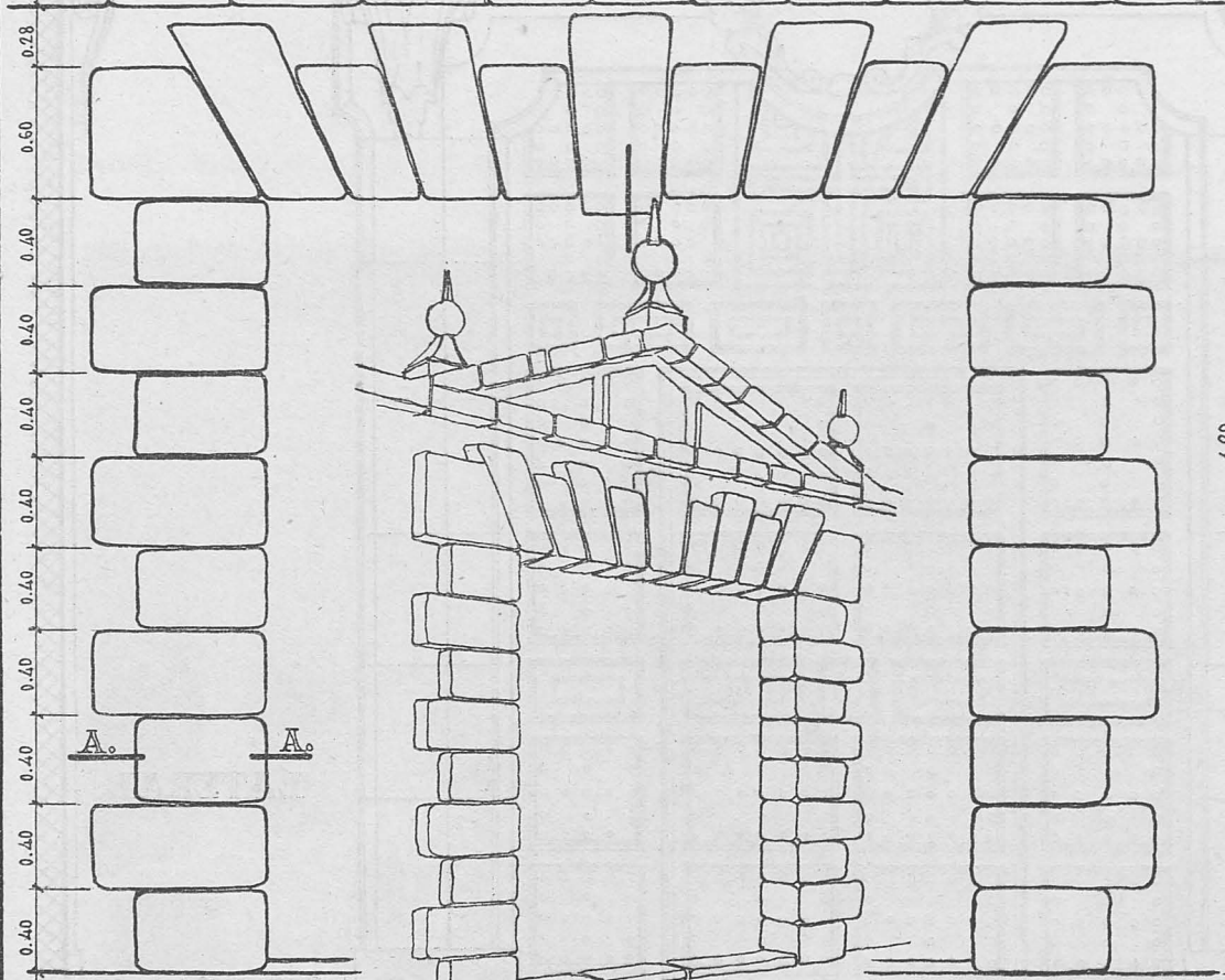
ALZADO.
