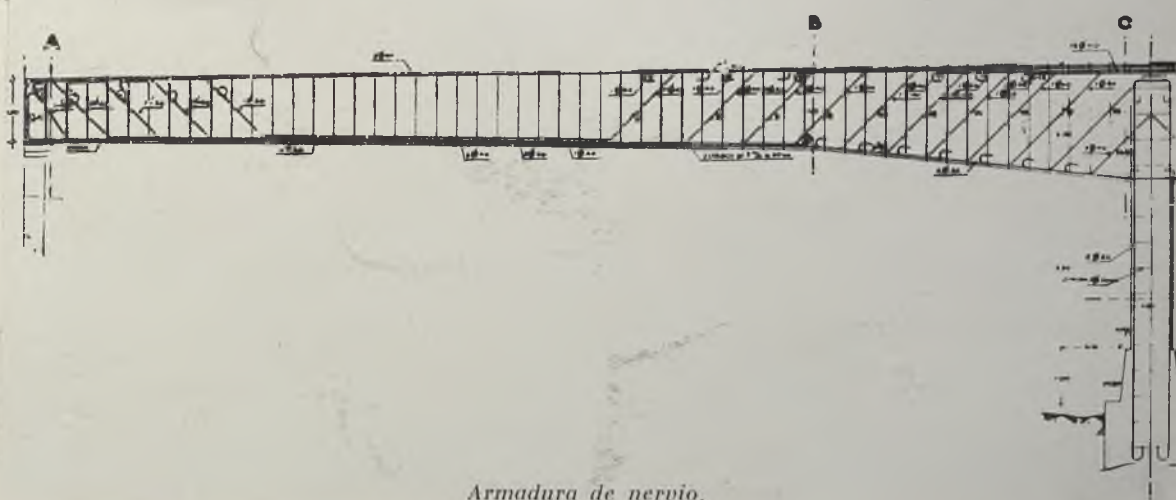
Armadura de nervio.
