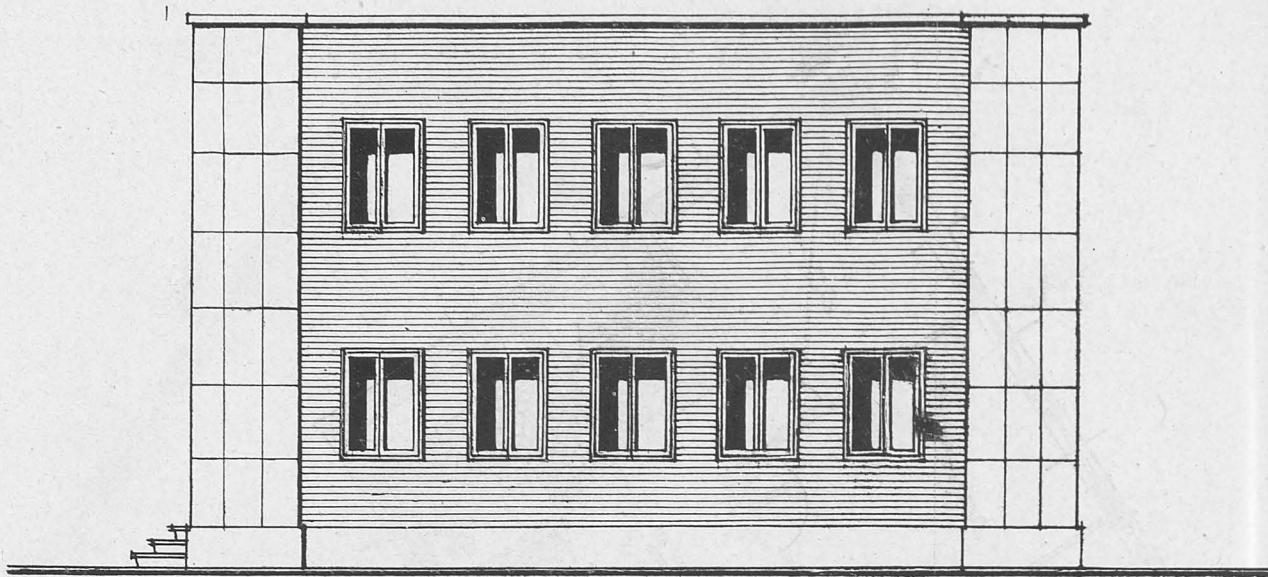
Fachada lateral.
