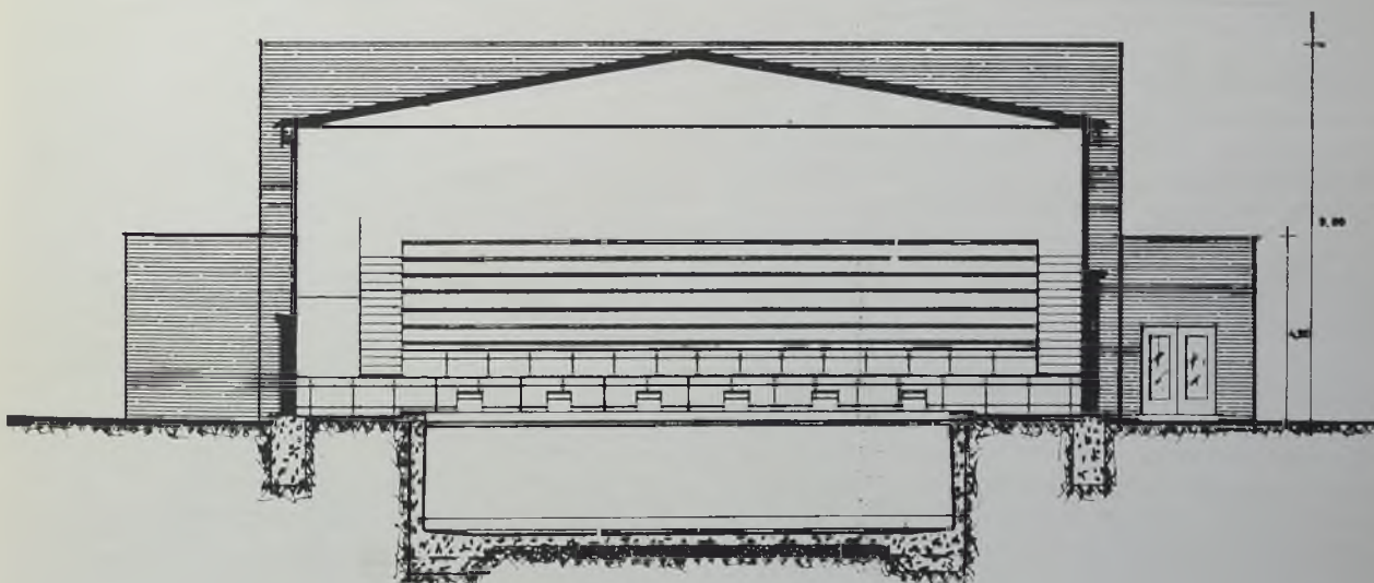
Corte frontal de la piscina cubierta con la tribuna de fondo.
